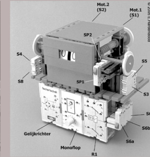
Telwerk 2 cijferig
